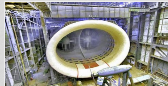
Металлоконструкции опорных мачт для аэродинамических труб. Центральный Аэрогидродинамический Институт г. Жуковский.
